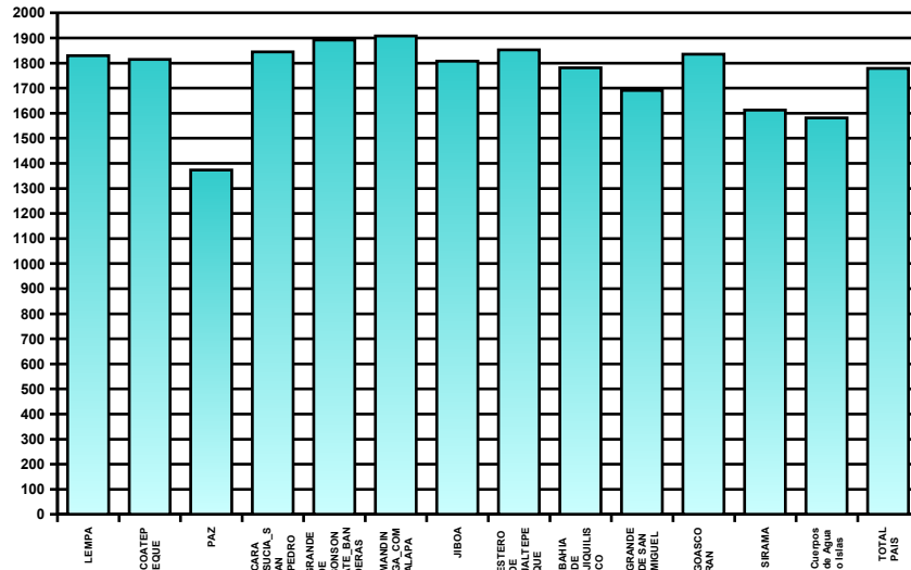
PRECIPITACION MEDIA ANUAL EN EL SALVADOR (mm)
