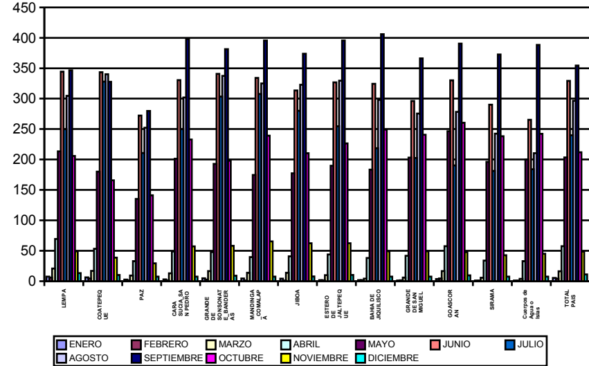
PRECIPITACION MEDIA MENSUAL EN EL SALVADOR (mm)
