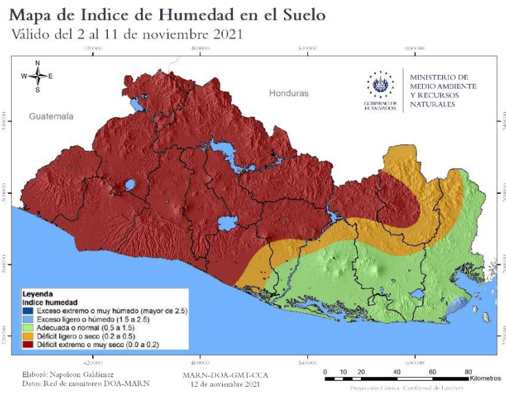
Figura 3. Mapa de Índice de humedad en el suelo entre el 02 y el 11 de noviembre 2021. Fuente: MARN-DOA-GMI-CCA
