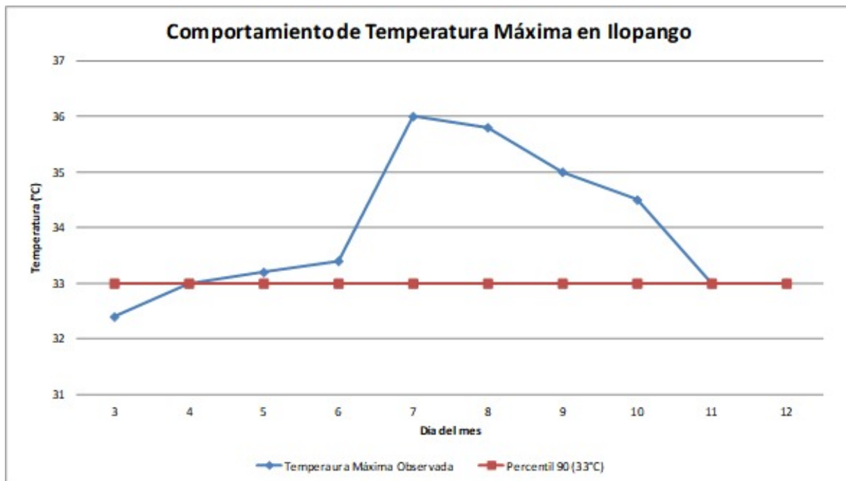
Figura 1. Registro de temperatura máxima en la estación meteorológica de Ilopango, para monitorio de la ola de calor
